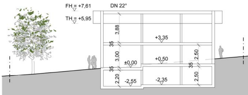
Längsschnitt Einfamilienhaus
